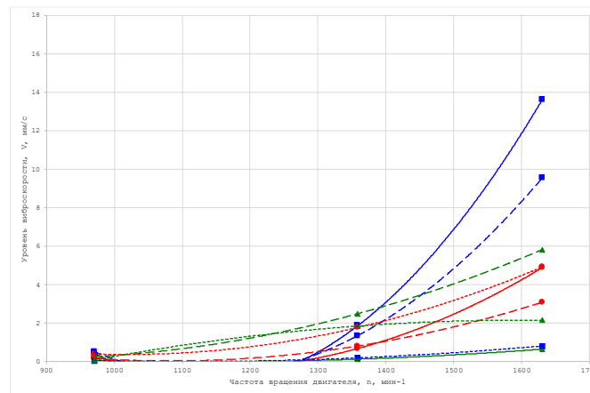
ГВРК плавкрана ПБ Уровни виброскорости на частоте 2-й гармоники
