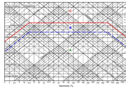
Нормы вибрации ГВРК согласно правил РМРС
