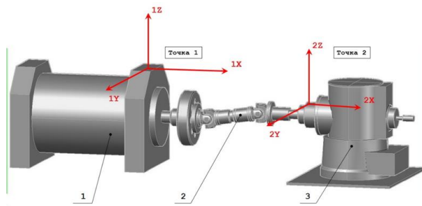
Схема проведения измерений на ГВРК с приводом от электродвигателя
