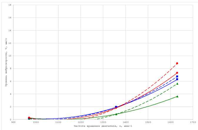
Электродвигатель плавкрана ПБ Уровни виброскорости на частоте 2-й гармоники
