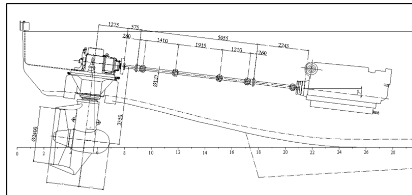
Валолиния с карданным валом
