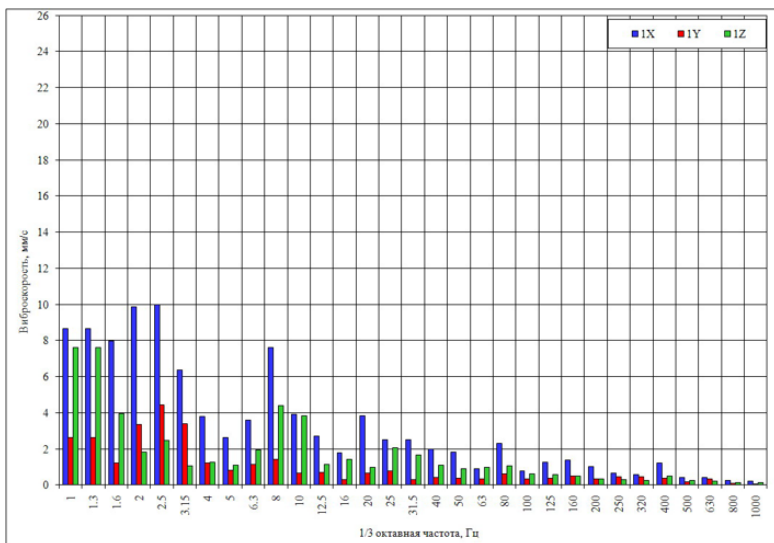
Валолиния без карданного вала
