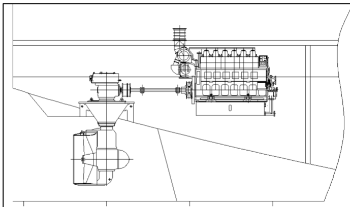
Валолиния без карданного вала
